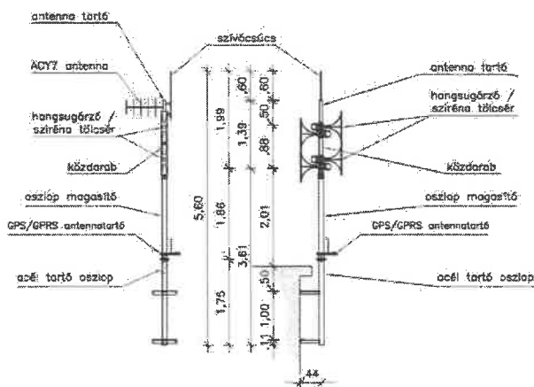
Összeállítási rajz körsugárzó elrendezés (ACY7 antenna) M=1:75
